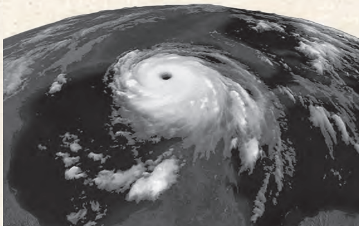
El huracán Katrina en el pico de intensidad, 28 de agosto de 2005, NASA.
